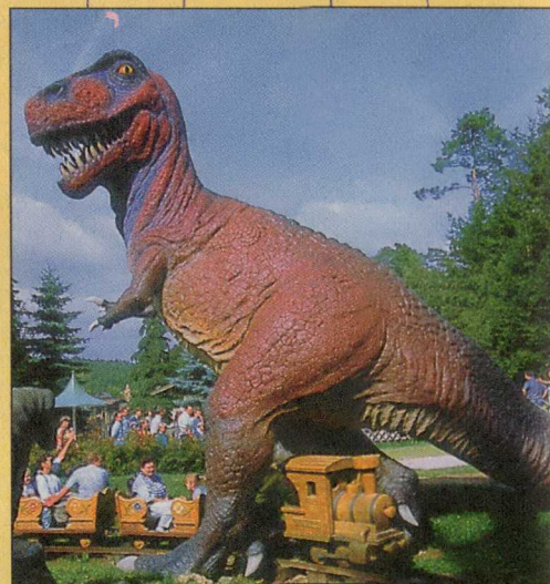
Mini-Eisenbahn
